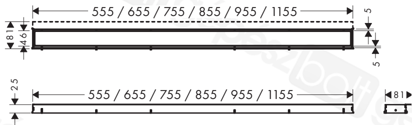
RainDrain Match 56036XXX - 56042XXX
